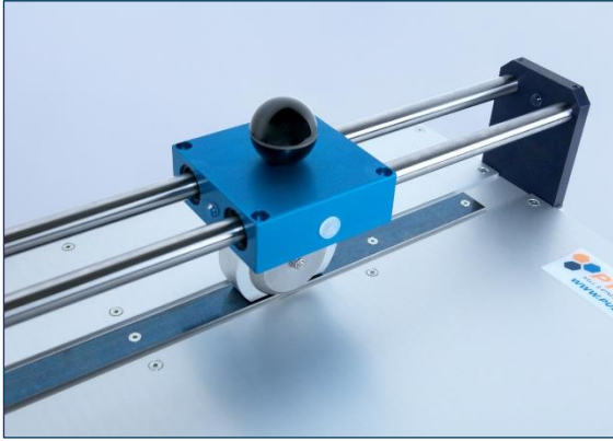
Wartungsfreie Messerführung
